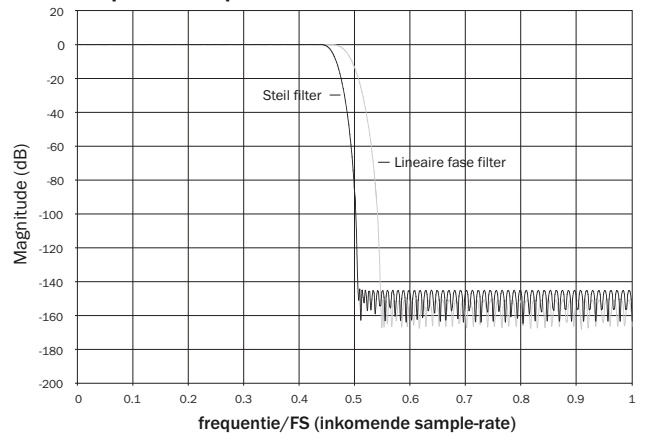
Frequentierespons steile filter
