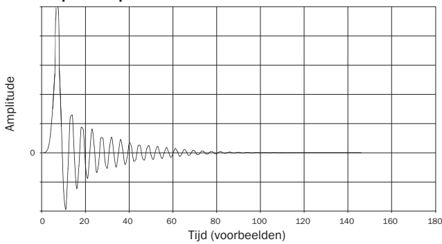
Impulsrespons minimale fase
