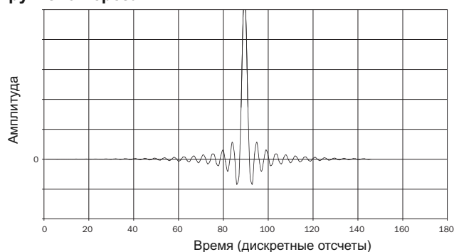
Импульсная характеристика фильтра с высокой крутизной среза
