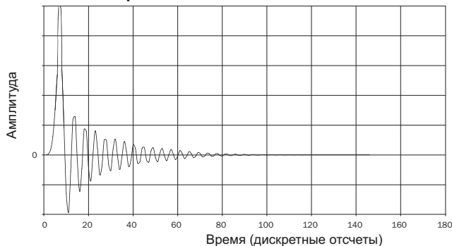
Импульсная характеристика фильтра с минимальной фазой
