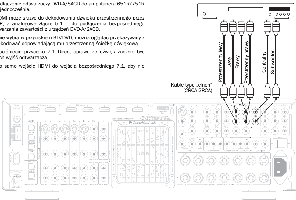
Odtwarzacz DVD-A lub wielokanałowy odtwarzacz SACD – podłączenia 5.1
