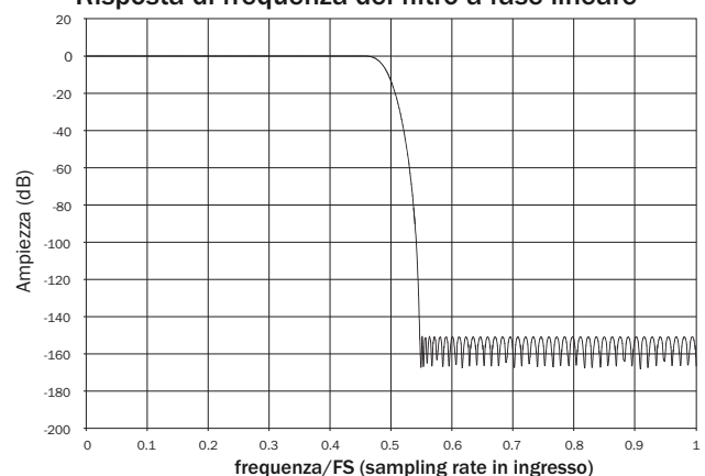
Risposta di frequenza del filtro a fase lineare
