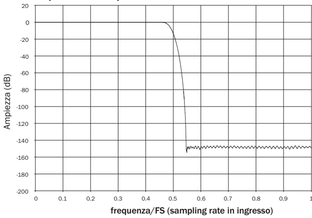
Risposta di frequenza del filtro a fase minima
