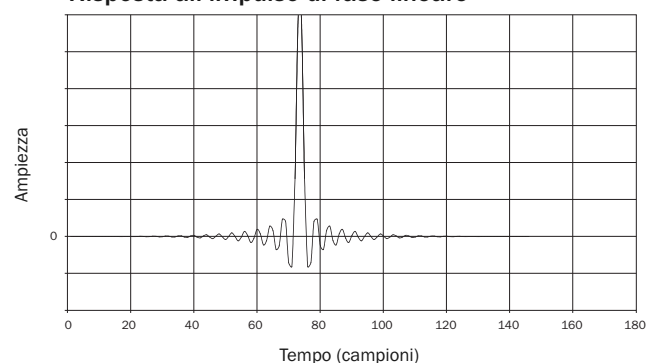
Risposta all'impulso di fase lineare
