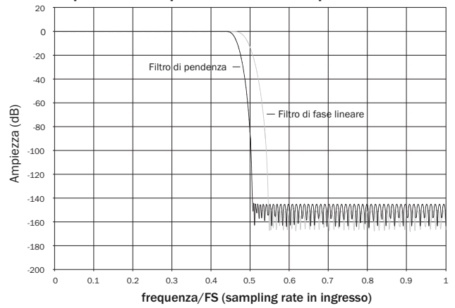
Risposta di frequenza del filtro di pendenza
