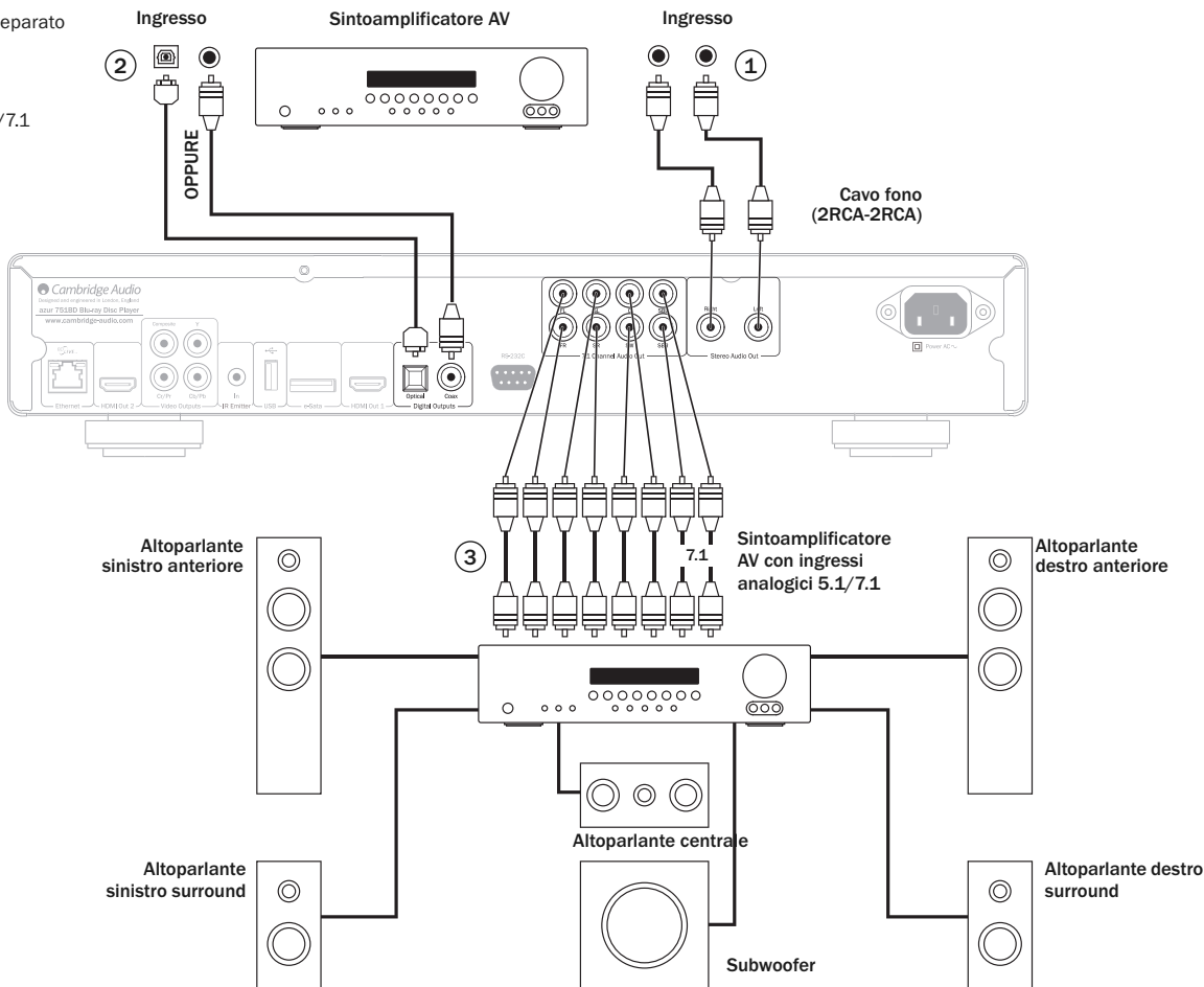
Illustrazione del diagramma degli altoparlanti per l'impostazione del canale 5.1. Per 7.1 aggiungere due altoparlanti posteriori.
