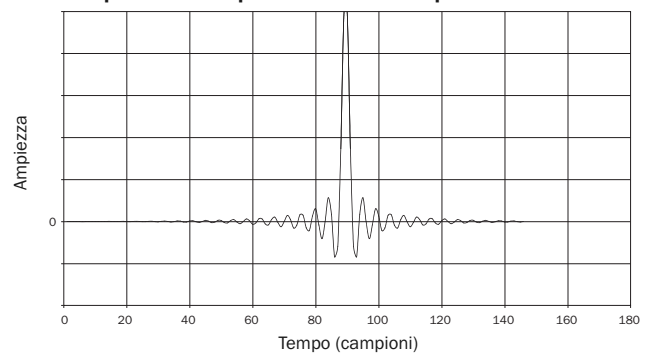
Risposta all'impulso del filtro di pendenza
