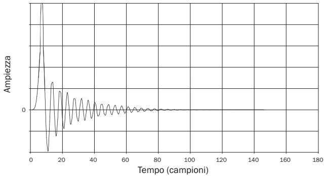
Risposta all'impulso a fase minima
